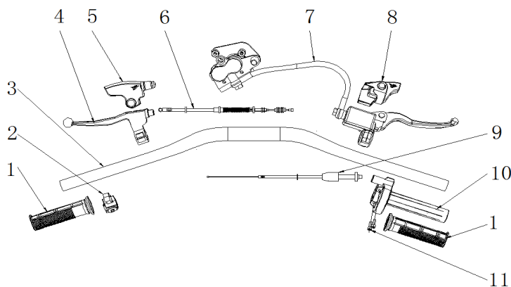
手把操纵件 HANDLE CONTROLLER
