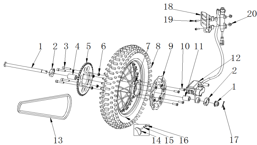
后轮/后制动器 RR.WHEEL/RR. BRAKE ASSY.
