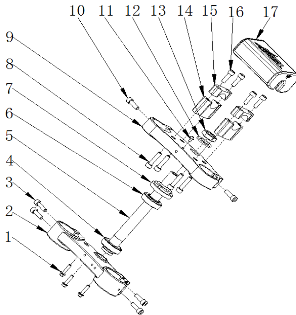
方向把/方向柱 HANDLE BAR/STEERING STEM
