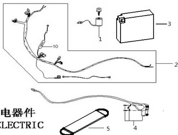
电器件(电启动) ELECTRIC (E-START)
