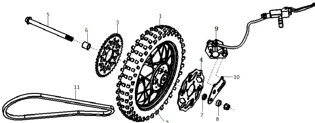
后轮/后制动器 RR. WHEEL/ BRAKE ASSY
