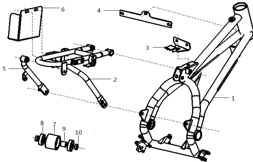
车架 FRAME
