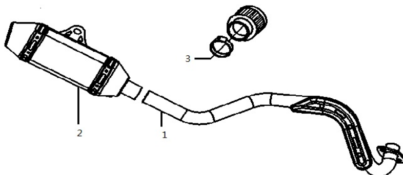
空滤器/排气消声器 AIR FILTER/MUFFLER
