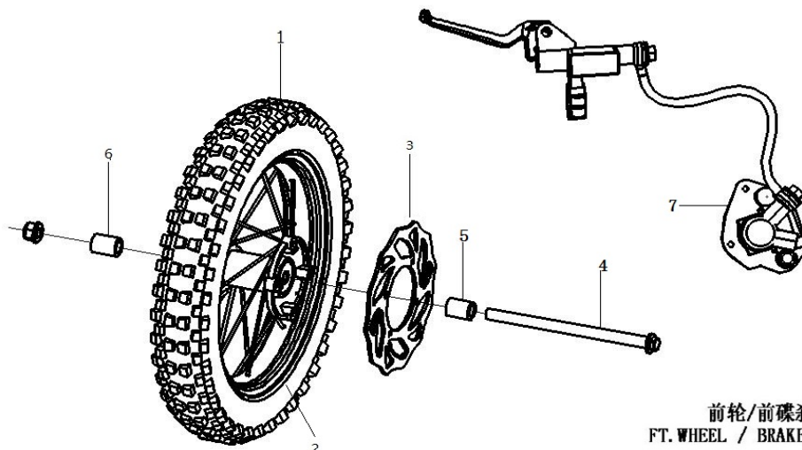
前轮/前碟刹 FR.WHEEL/FR.BRAKE ASSY.
